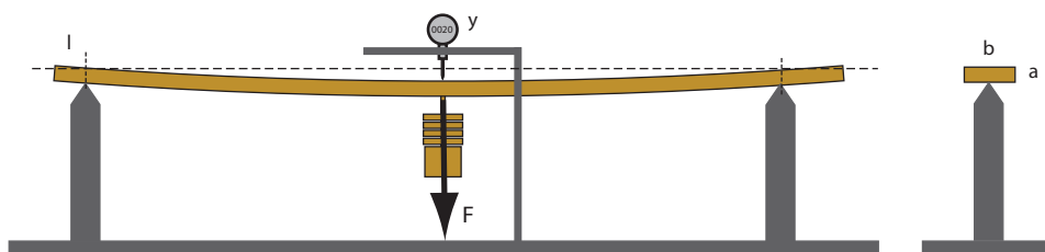
Obrázek 4: Průhyb nosníku
