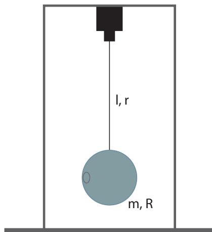
Obrázek 5: Torzní oscilátor
